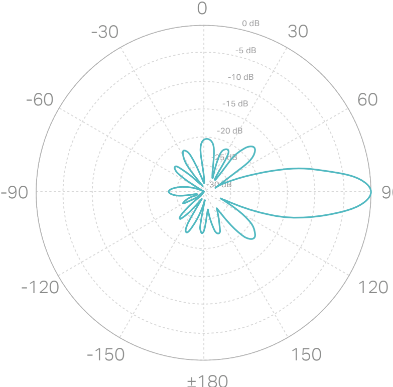
Elevation
